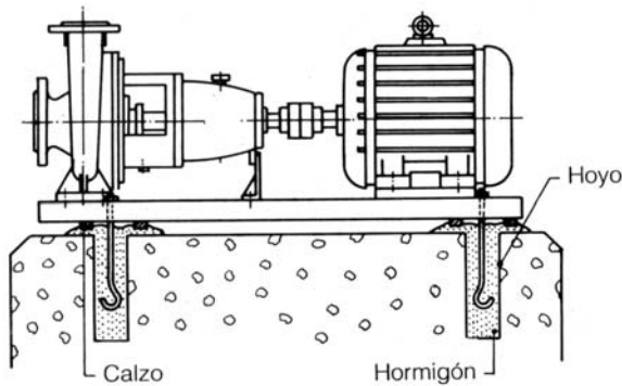
Fig. 4 – Asentamiento de la base
