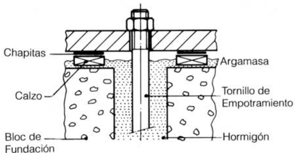
Fig. 5 – Nivelación de la base
