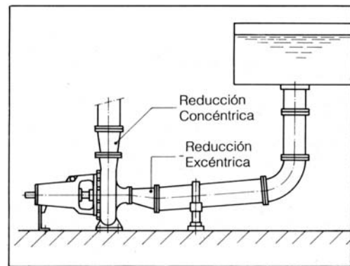
Fig. 11 – Aspiración positiva
