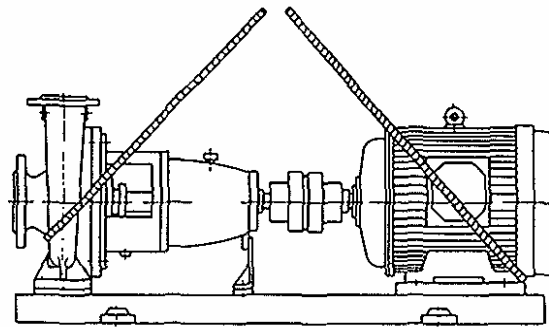
Fig. 3 – Transporte del conjunto motobomba
