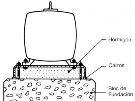
Fig. 6a – Llenado de la base con Hormigón
